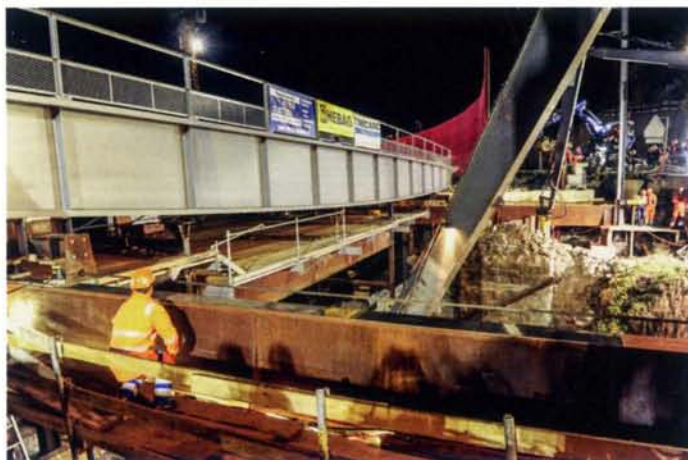
Die massiven Stahlträger mit ihren Gleitflächen für den Brückenverschub.
